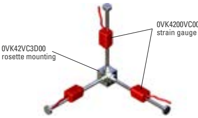
Extensómetros en configuración en 3-D
