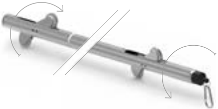
Espir l metro: sonda para medir la torsi n respecto al eje de la tuber a inclin m trica.
